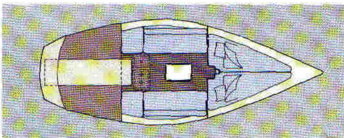
Die großzügige großzügige Geräumig- keit der Kajüte wird unter- durch den freien ing zu der breiten dekoje im Vorschiff. dies eine Folge des in Kiels, der die aufwen- und platzgreifende Hub- mechanik überflüssig macht.
